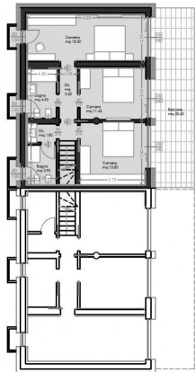
Pianta piano terra - scala 1:100
