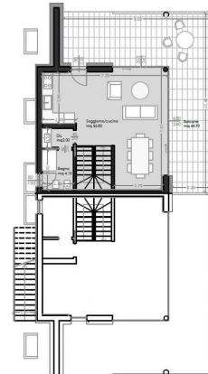
Pianta piano primo - scala 1:100
