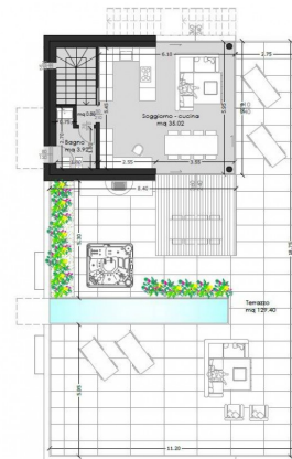
Pianta piano copertura - scala 1:100
