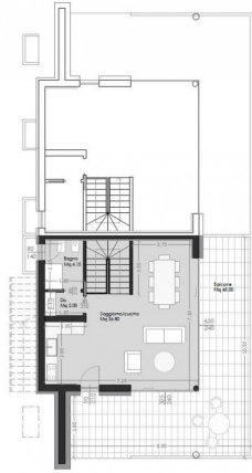
Pianta piano primo - scala 1:100
